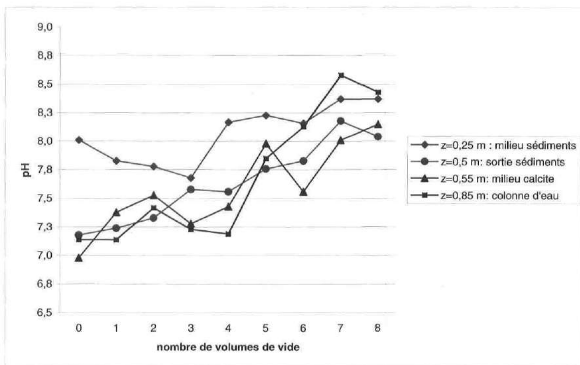
Figure 5.8: Variation du pH pour la colonne A (avec alun)
