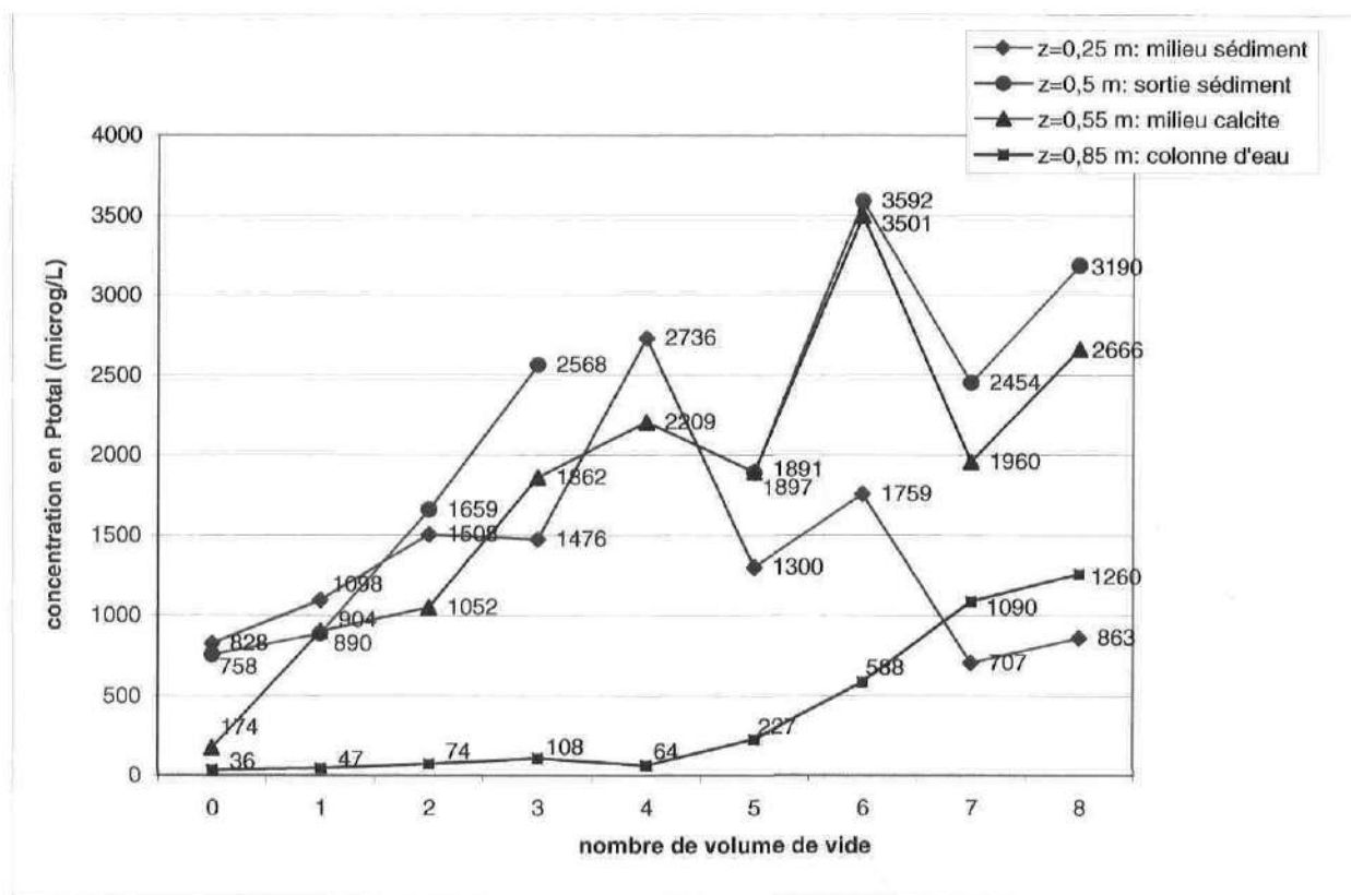
Figure 5.14: Variation de la concentration en phosphore total dans la colonne A (avec alun)
