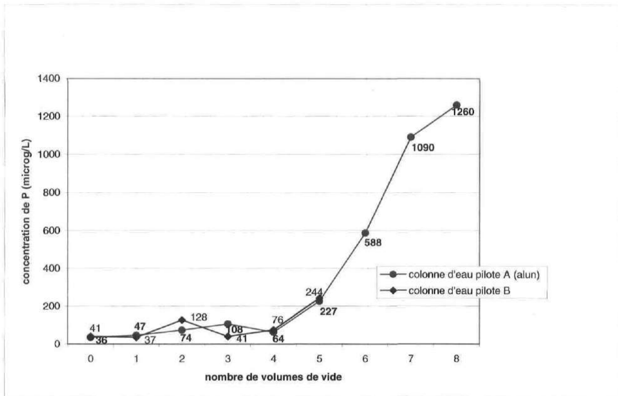
Figure 5.16: Comparaison entre les deux essais en colonnes pour la concentration en P dans la colonne d'eau ( z=0,85 m)
