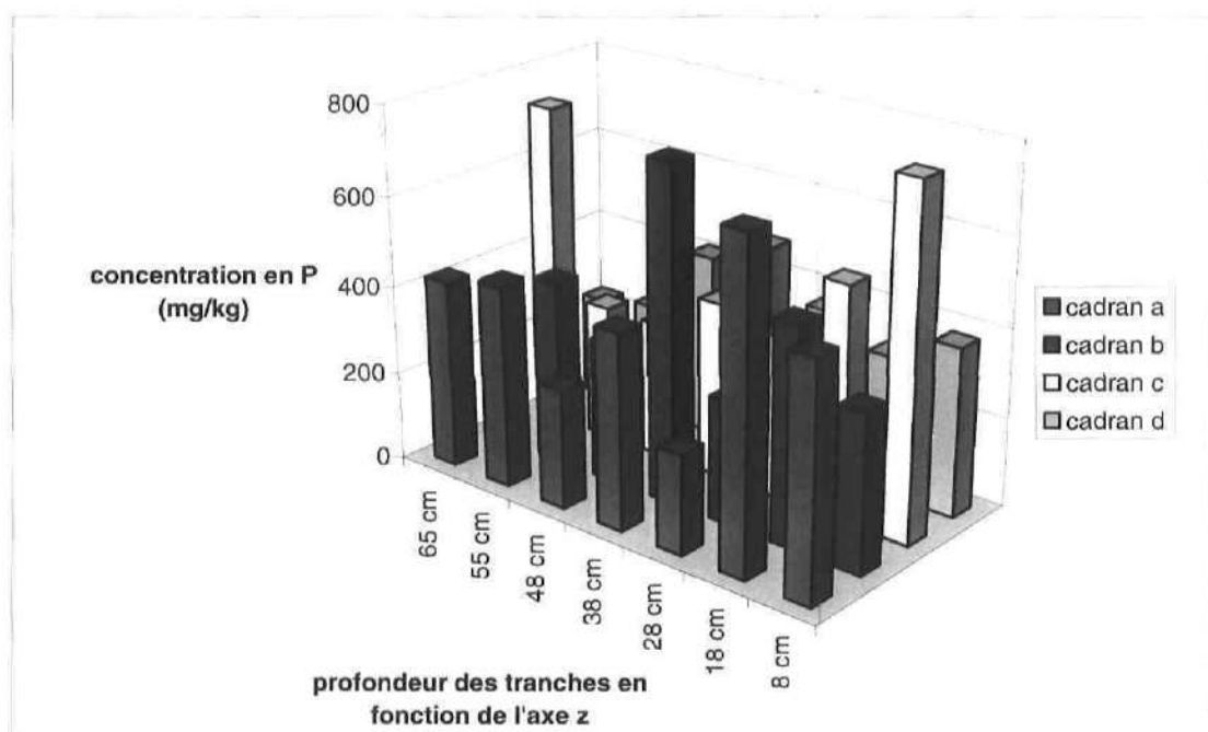
Figure 5.20 : Variation de la teneur en phosphore dans les couches pour chaque tranche et cadran (colonne B)
