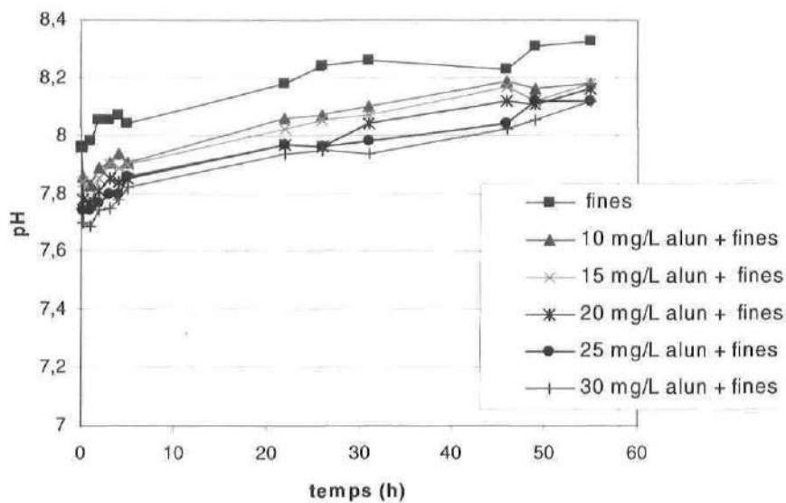
Figure 5.4 : Évolution du pH pour la série avec alun et calcite fine
