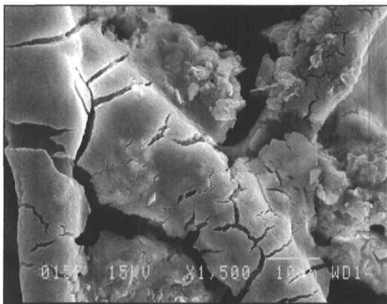
Figure 5.6 : hydroxyde d'aluminium au MEB
