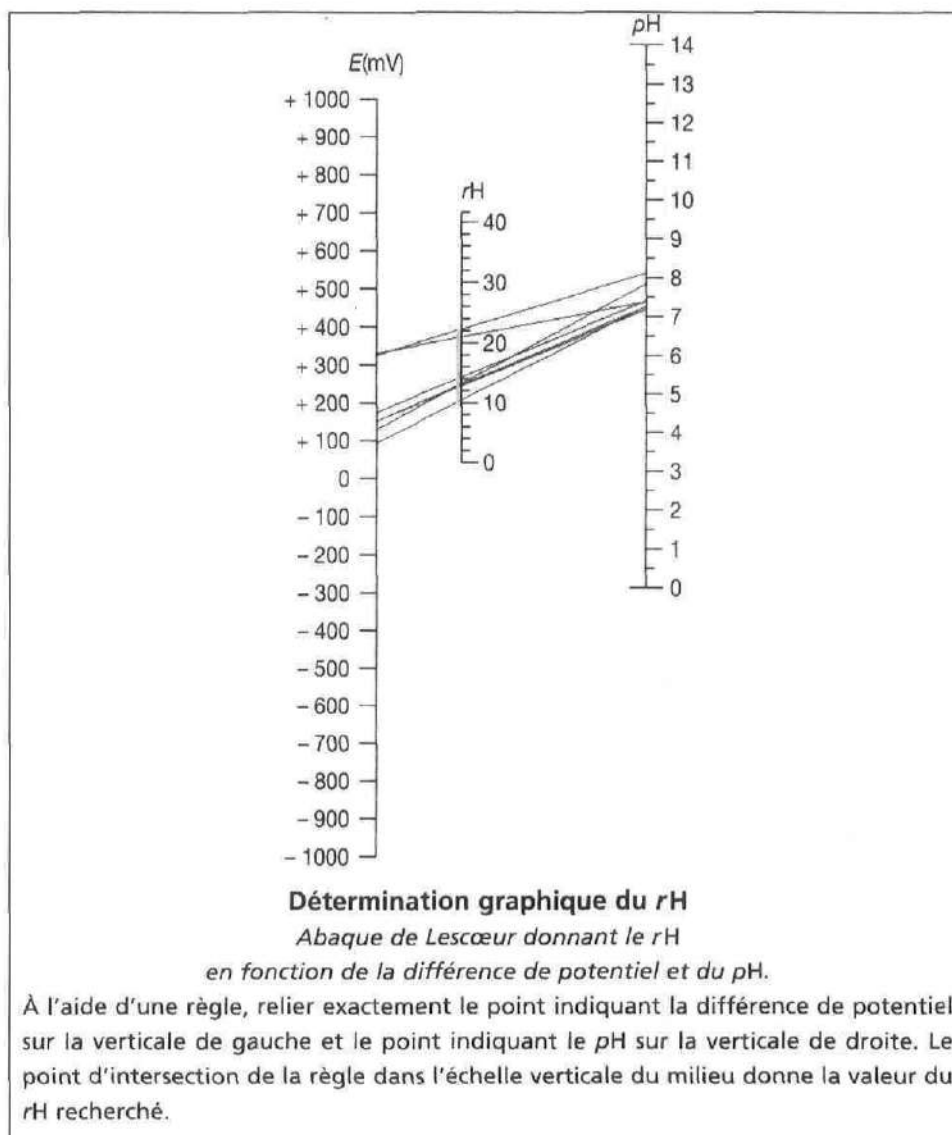
Figure 5.13 : Détermination du pouvoir d'oxydo-réduction rH (tiré et adapté de Rodier et al., 1996)
