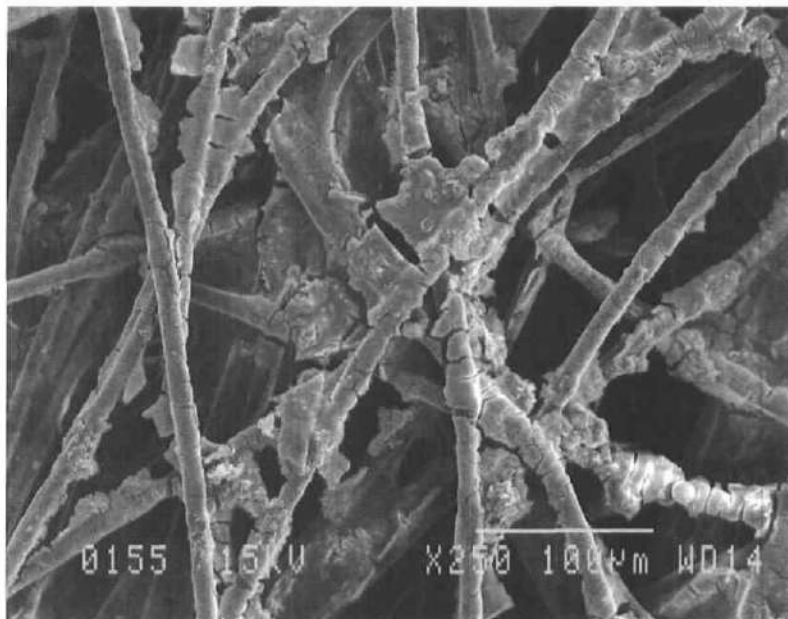
Figure 5.5 : photographie du filtre au MEB
