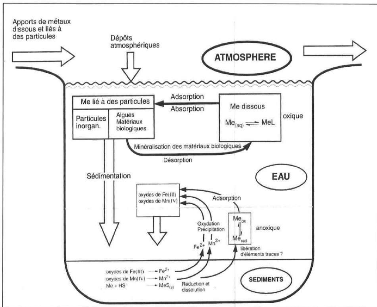
Figure 3.1 : Schéma des processus qui déterminent les concentrations des métaux dans la colonne d'eau d'un lac (tiré de Sigg et al., 2000)
