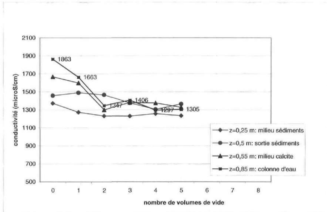
Figure 5.11: Variation de la conductivité dans la colonne B
