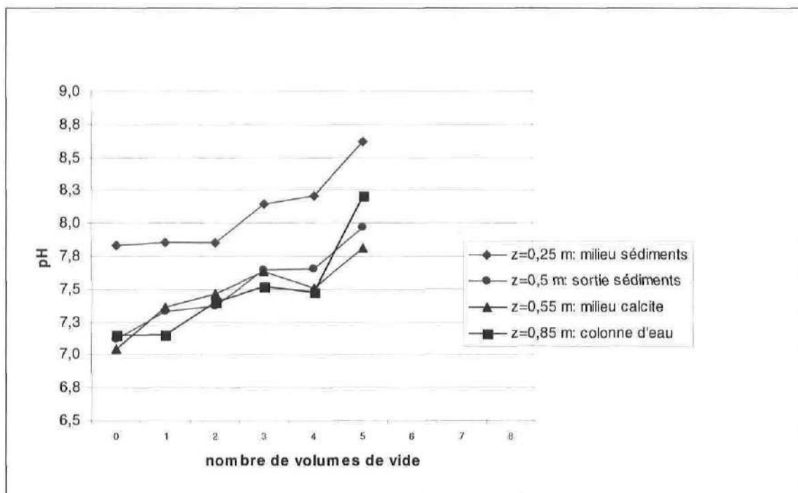
Figure 5.9 : Variation du pH pour la colonne B
