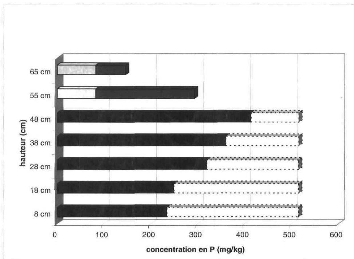
Figure 5.19: Répartition du phosphore dans les couches de la colonne A en fonction de la profondeur
