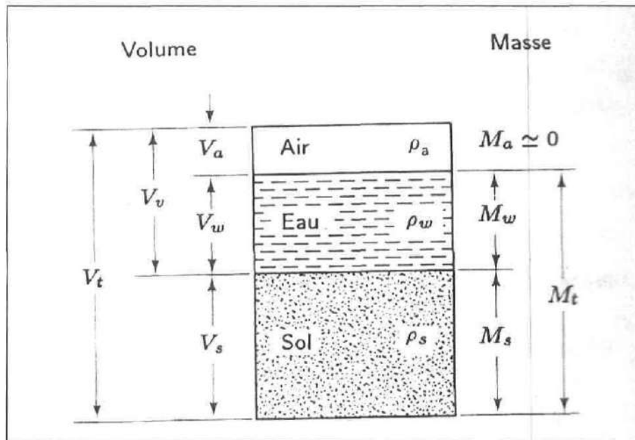
Figure A4-2 : Diagramme de phase (tirée de Holtz et Kovacs, 1991)
