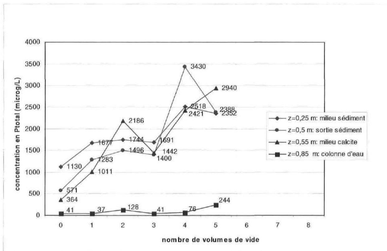
Figure 5.15: Variation de la concentration en phosphore total dans la colonne B
