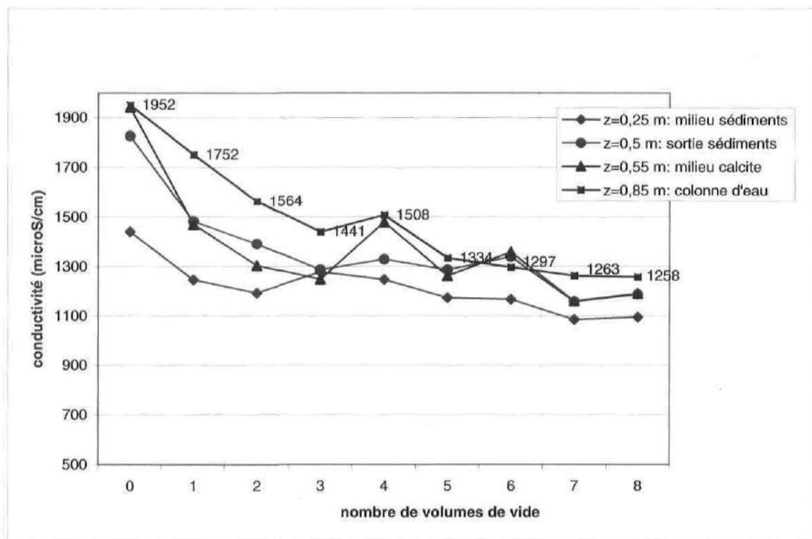
Figure 5.10: Variation de la conductivité dans la colonne A (avec alun)
