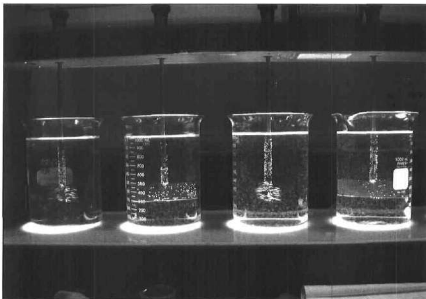
Figure 4.3 : Essai en "jar test" (série 1)
