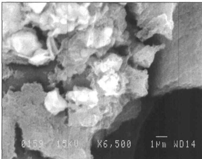
Figure 5.7 : Hydroxyde de fer et de manganèse au MEB
