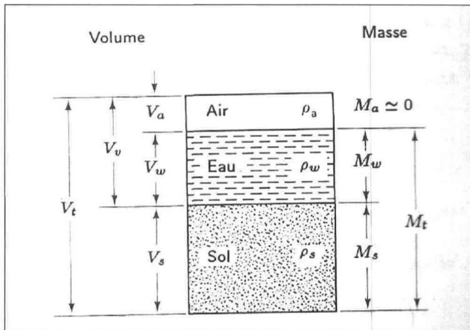
Figure 4.9 : Diagramme de phases (tiré de Holtz et Kovacs, 1991)
