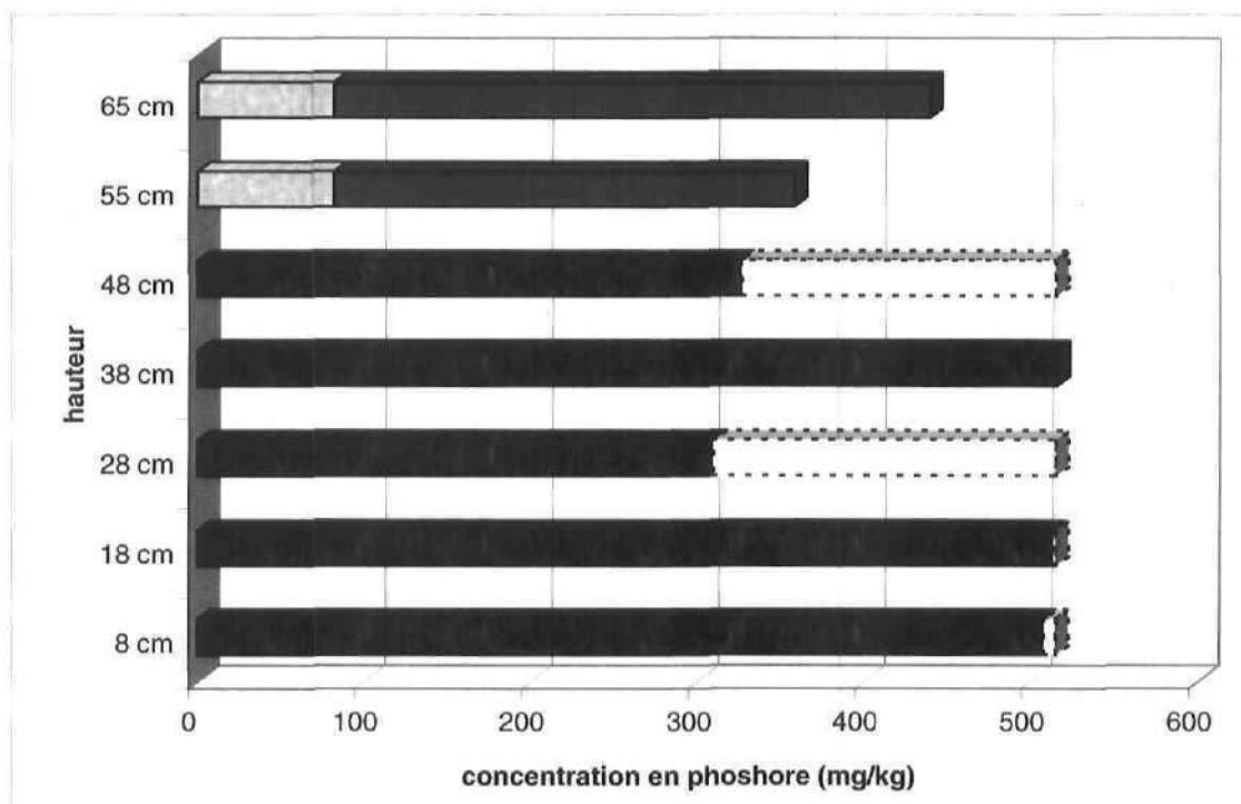
Figure 5.21 : Répartition du P dans les couches de la colonne B en fonction de la profondeur
