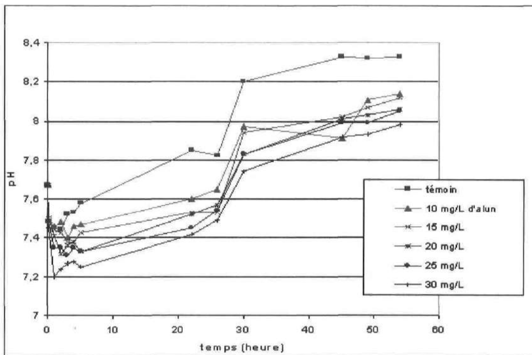
Figure 5.2 :  volution du pH pour l'alun seul
