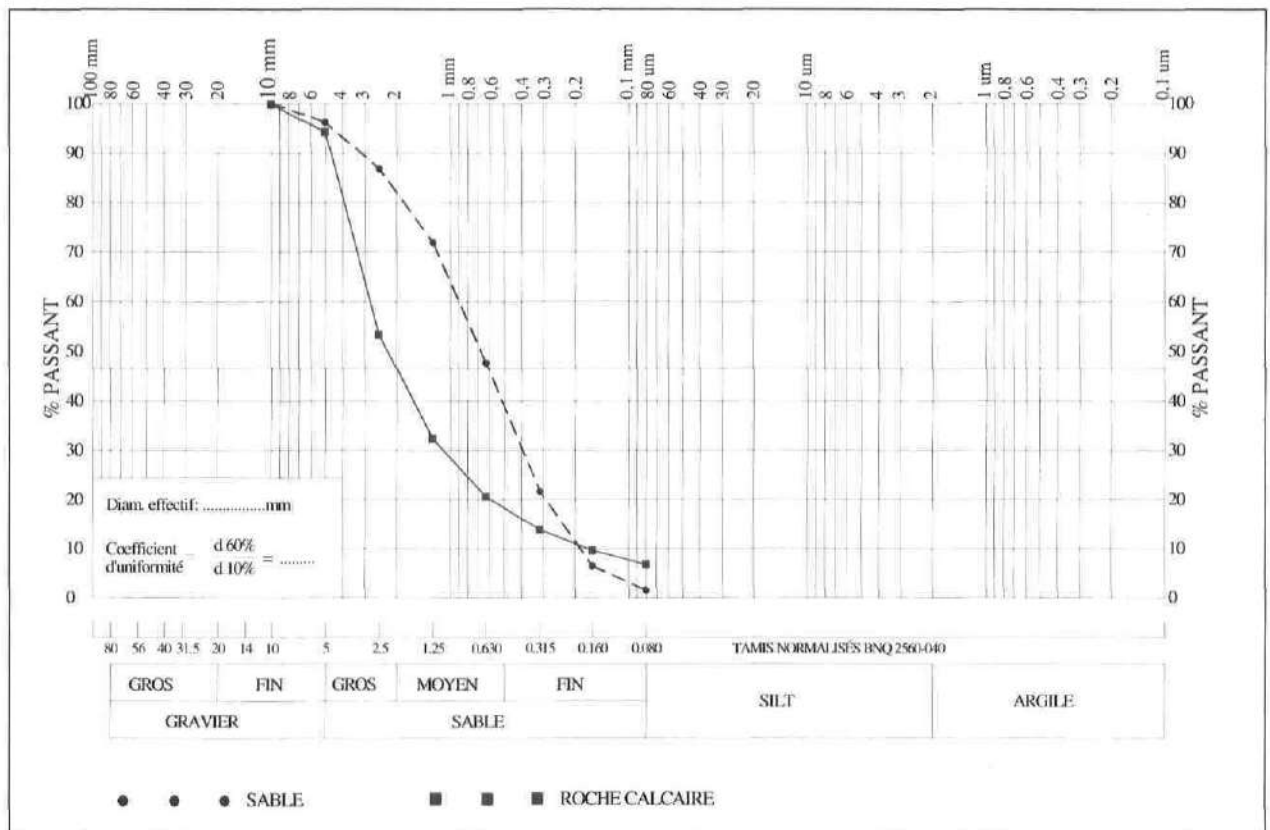
Figure 4.2 : Courbes granulométriques de la roche calcaire et du sable (tiré de Dominguez, 2004).
